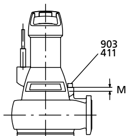
Рис. 19: Долив смазочной жидкости
